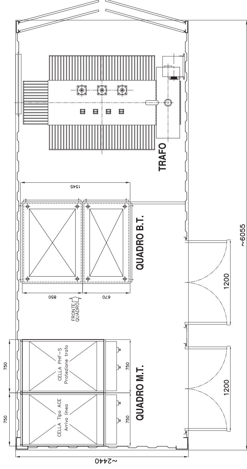
VISTA IN PIANTA DISPOSIZIONE APPARECCHIATURE INTERNE
