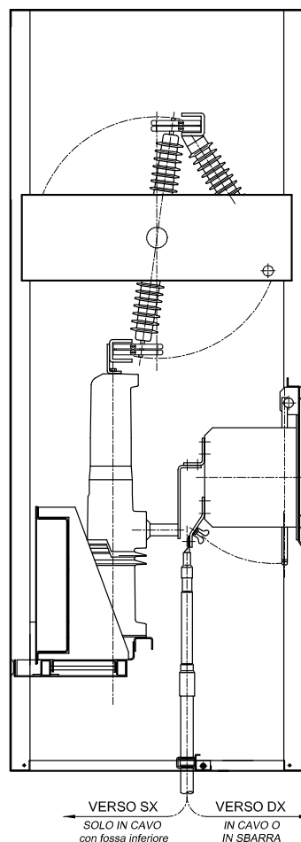
SEZIONE INTERNA
