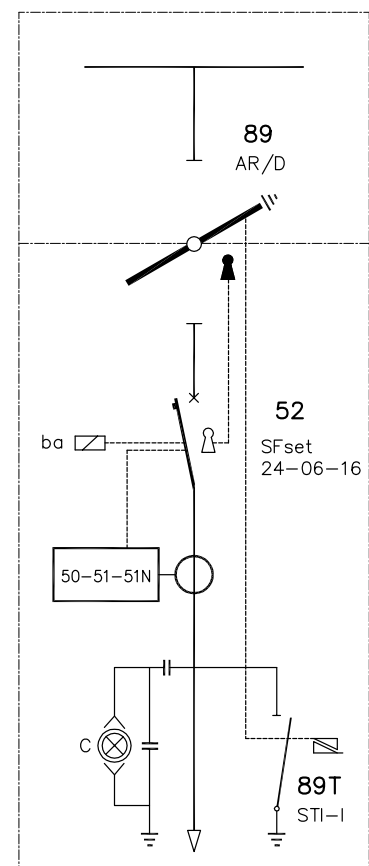
SCHEMA UNIFILARE
