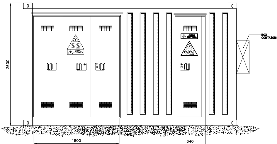
FRONTE ESTERNO CABINA
