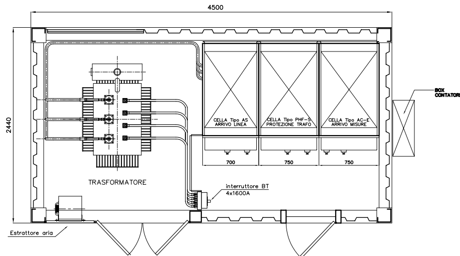
PIANTA INTERNA CABINA
